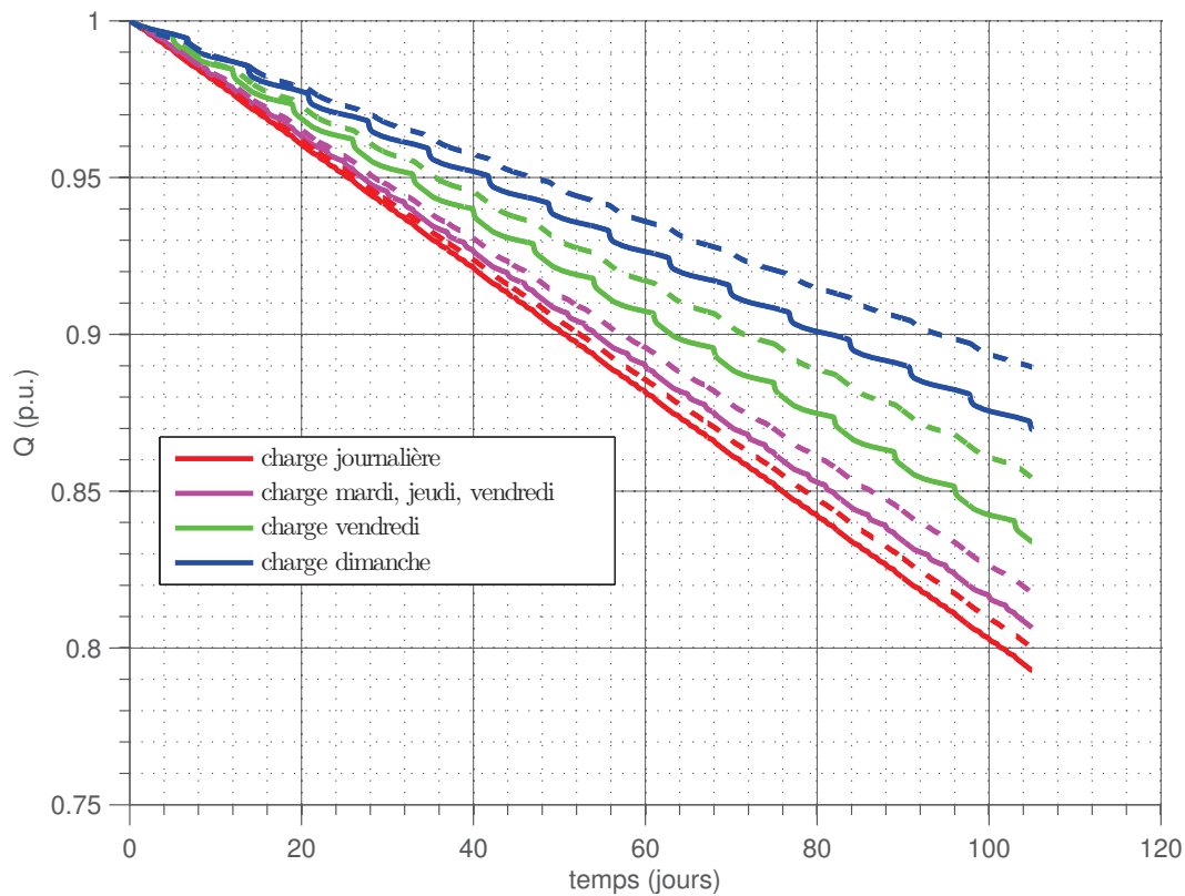
FIGURE 5.14. Simulations pour les quatre stratégies de charge d'un véhicule (exemple 1). Sur la figure les courbes en traits tiretés représentent les évolutions sans prise en compte des alternance de SoC , c'est-à-dire avec le modèle de vieillissement uniquement calendaire ; les courbes en traits continus représentent les évolutions du modèle avec prise en compte des alternances de SoC .
