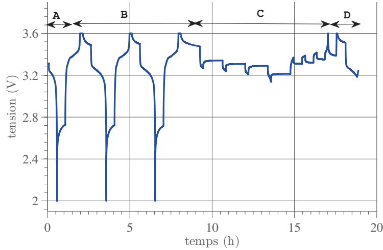
FIGURE 4.7. Profil de tension d'une cellule LFP lors d'un RPT SIMCAL.
