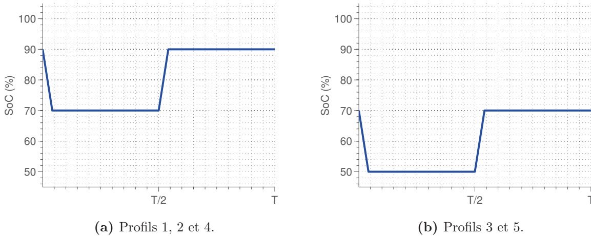
FIGURE 4.13. Schéma des profils d'alternance de SoC de la campagne LFP. Les profils 1, 2 et 3 se réalisent avec une charge en CCCV ; les profils 4 et 5 se réalisent à courant constant (CC) en charge comme en décharge. Le régime de courant est C/2 pour le profil 1 et C/5 pour tous les autres profils.
