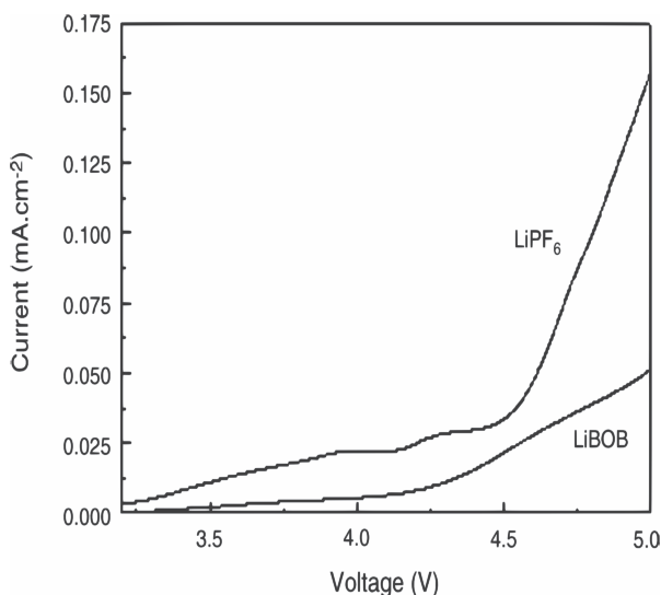
(d) Courbes de courant-potentiel pour \text{LiPF}_6 et \text{LiBOB}
