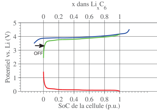
(d) LR = 80 \% , OFF = 10 \%
