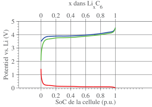
(a) Cellule parfaitement équilibrée ( LR = 100 \% , OFF = 0 \% )
