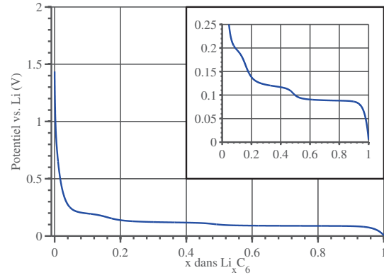
(b) Potentiel du graphite versus Li, approximation numérique [80] à partir des mesures de [81].
