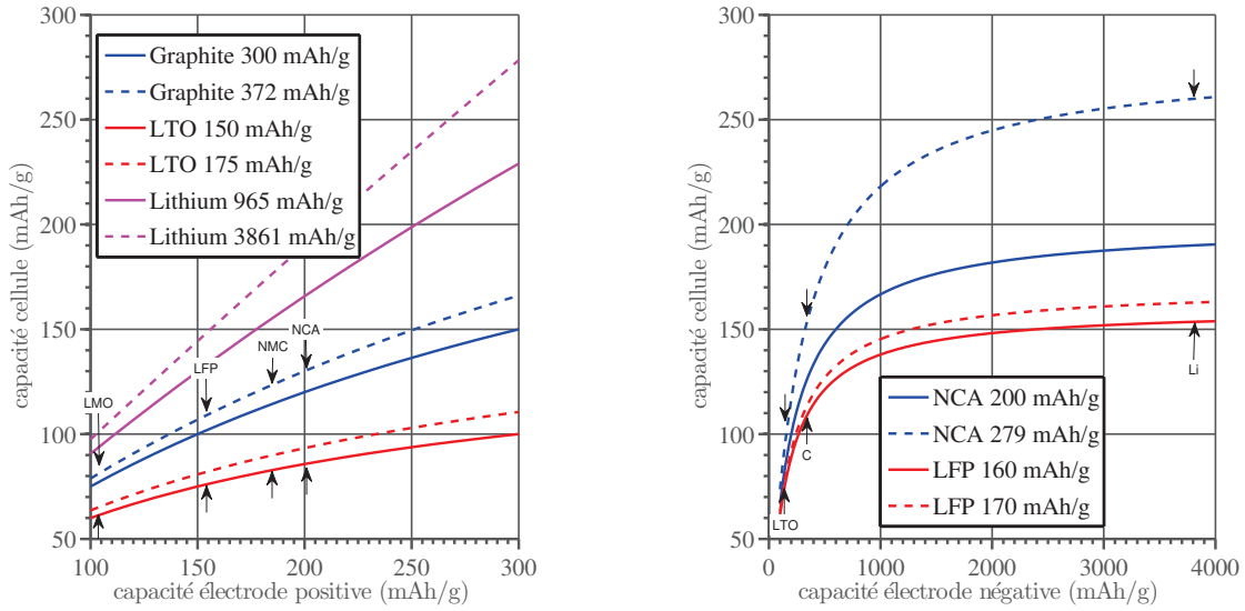
(a) Variation en fonction de la capacité spécifique de la positive pour plusieurs électrodes négatives. Traits continus : capacités réelles, traits tiretés : capacités théoriques (maximum atteignable) (b) Variation en fonction de la capacité spécifique de la négative pour plusieurs électrodes positives. Traits continus : capacités réelles, traits tiretés : capacités théoriques (maximum atteignable)
